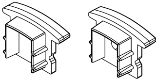
End Cap (Pair) #EC
